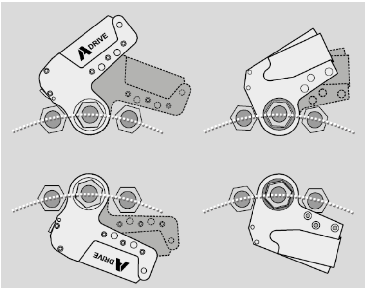
Abbildung 1: Das patentierte Design des Sechskantantriebs sorgt für längste Reichweite. So passt der Sechskantkopf ohne Rütteln oder manuelles Einrichten der Ratsche einfach auf die Mutter.
